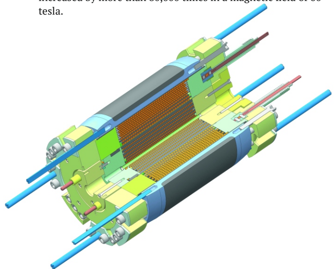
Fig. 2: Konstruktionskizze einer Hochfeld-Magnetspule zur Erzeugung von gepulsten Magnetfeldern. // Construction sketch of a high magnetic field coil for the generation of pulsed magnetic fields. (© HZDR)
